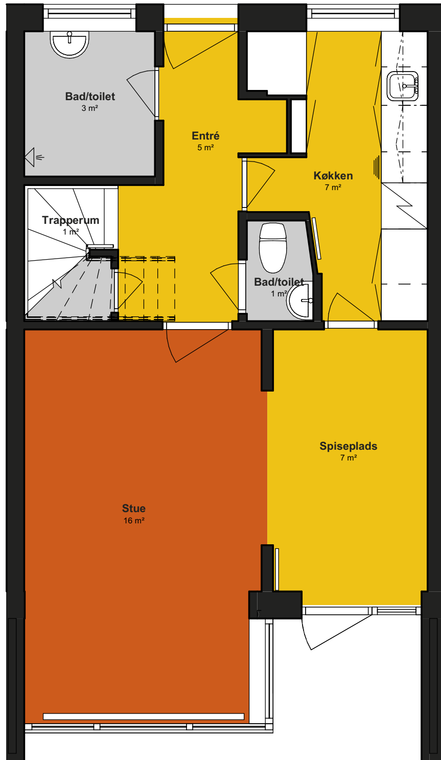
Stueplan
